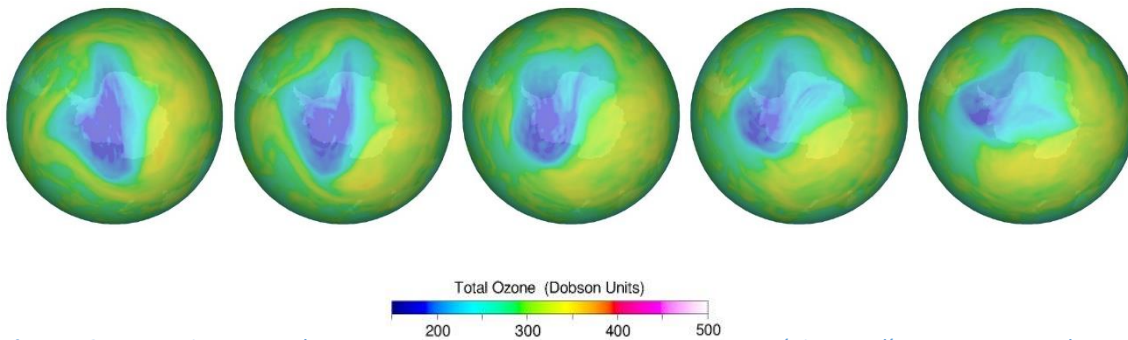
Figura 12. Proyecciones para los próximos 5 días que muestran la evolución y crecimiento del agujero de ozono.
