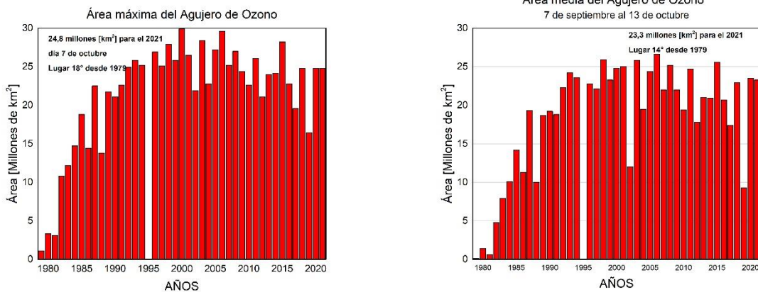
FIGURA 11. ÁREAS MÁXIMAS PARA EL AGUJERO DE OZONO 2021.
