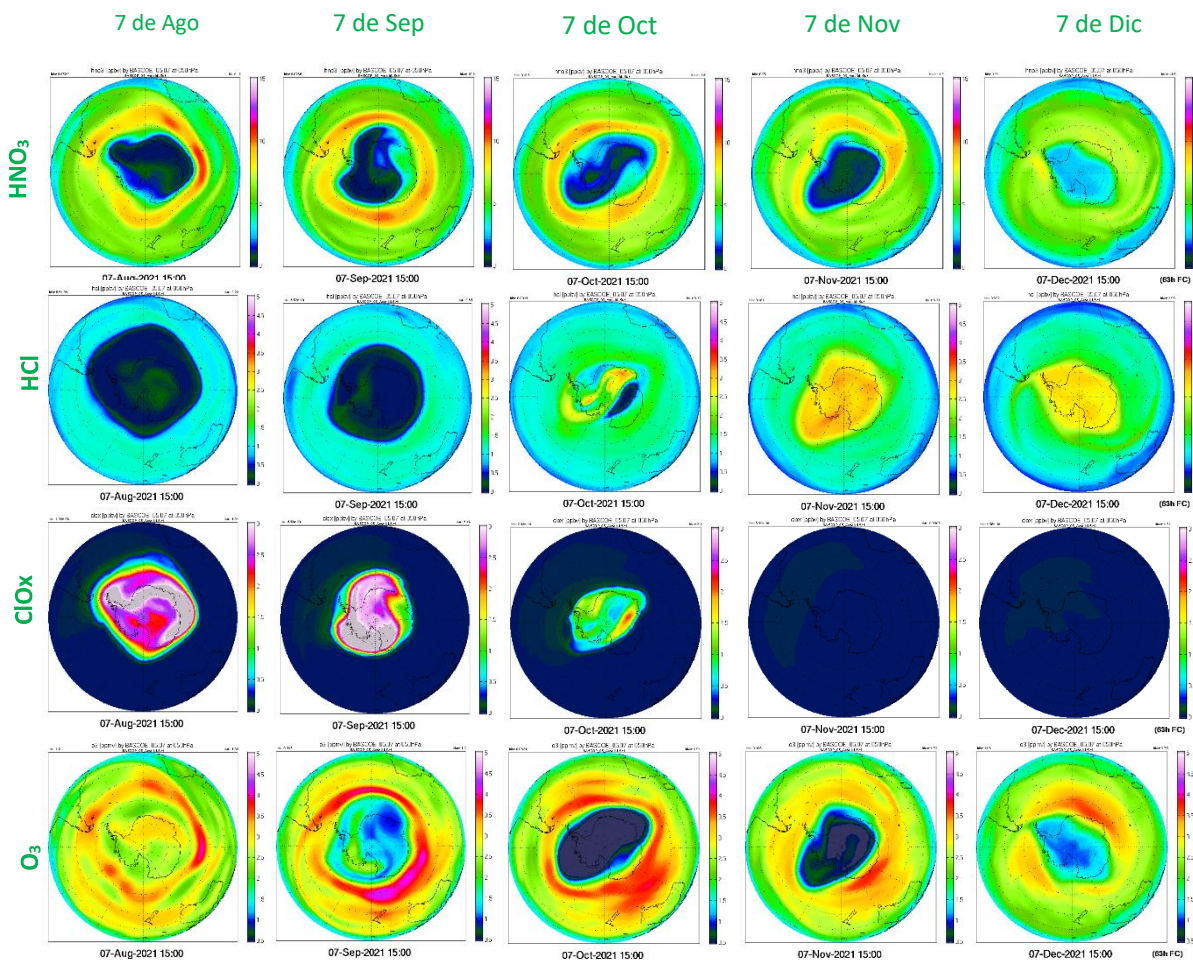
Figura 10. Resultados del modelo de asimilación BASCOE a 50 hPa. Este modelo se usa como parte del proyecto macc-II, ahora el NRT Análisis de ozono y especies relacionadas con el ozono. La primera fila muestra la relación de mezcla del ácido nítrico ( \text{HNO}_3 ). La segunda fila muestra la relación de mezcla para el ácido clorhídrico (HCl). La tercera fila muestra la relación de mezcla para el óxido de cloro y su dímero ( \text{ClOx} = \text{ClO} + (\text{ClO})_2 ). La última fila (abajo) muestra la relación de mezcla del ozono.
