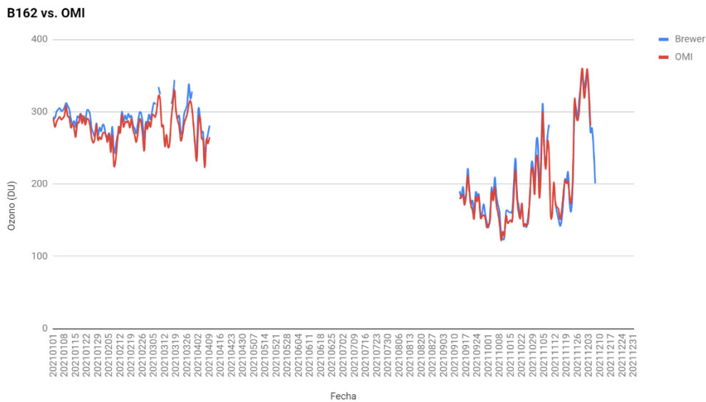
Registro (año 2021) del espectrofotómetro Brewer #162 vs el registro satelital de OMI en Base San Martí..
