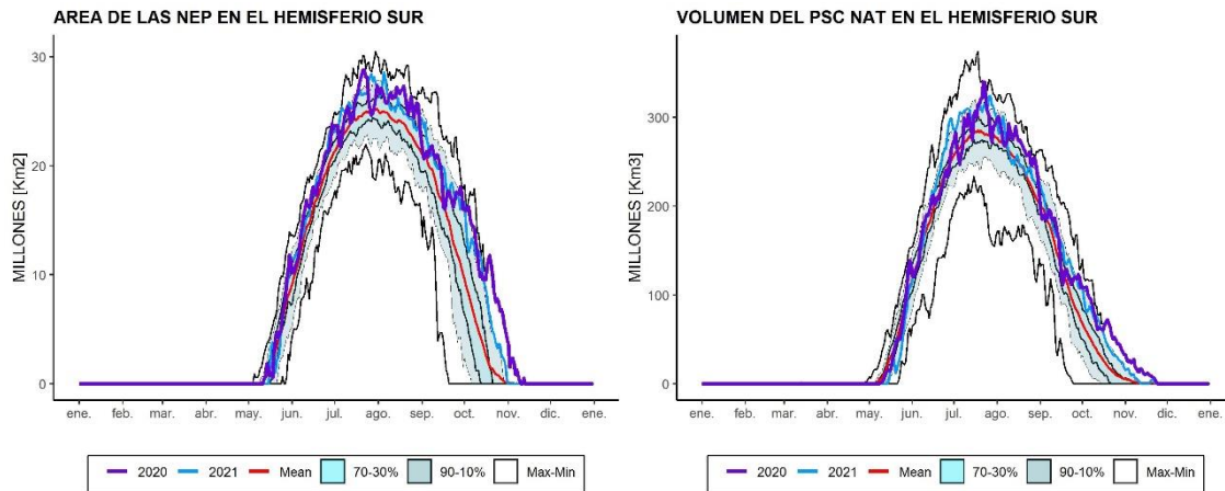
Figuras 2. Área de las nubes estratosféricas polares (NEP), sobre la región Antártica. La serie de tiempo donde las temperaturas están suficientemente bajas para la formación de las NEP Tipo I (ácido nítrico, trihidratado, -78,5^{\circ}\text{C} ) en el nivel isentrópico de 460 K. La línea color roja, representa la evolución del tamaño de las NEP para el año 2021 hasta el día 16 de noviembre (Ya no producen más NEP). La línea negra representa la media, la línea azul fuerte la media de 1979 a 2019. Las líneas externas negras, son los máximos y mínimos durante el periodo 1979 – 2019. Las líneas sombreadas en azul de adentro hacia fuera, son los percentiles de 70 – 30% y de 10 – 90%.
