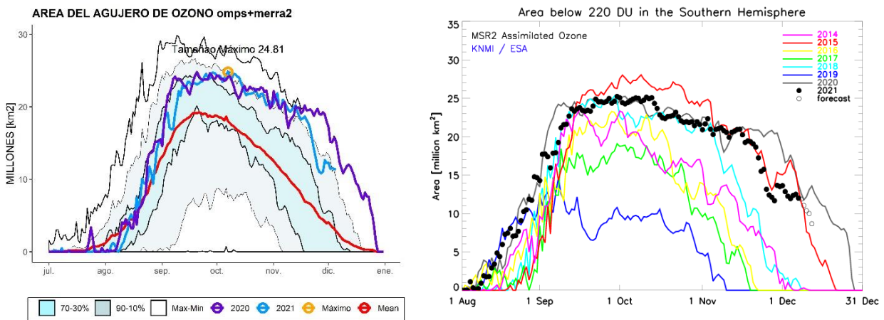
Figura 11. Área (millones de km 2 ) donde la columna total de ozono es menos de 220 unidades Dobson, hasta el 4 de septiembre. Izquierda; Satélites de la NASA, EEUU (TOMS+OMI+OMPS). Derecha, Datos de la ESA (Agencia Espacial Europea).
