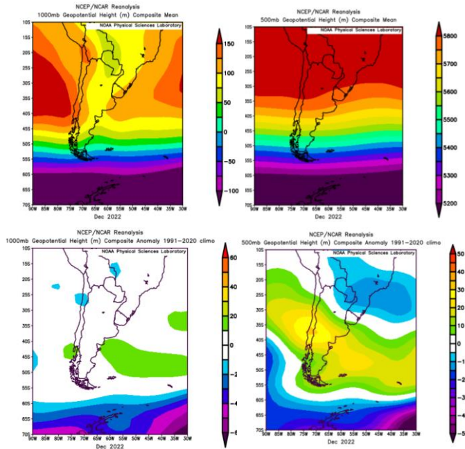
FIG.7– Campo medio de altura geopotencial de la superficie isobárica de 1000 y 500 hPa (arriba) (mgp) y anomalía (abajo) diciembre de 2022
