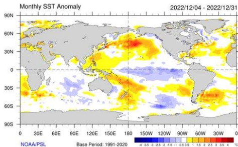
Figura 1 - Anomalías de la temperatura superficial del mar de diciembre de 2022. Período de referencia 1991-2020. Fuente: NOAA-CIRES/CDC
