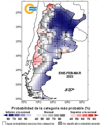
Pronóstico de Temperatura Media (Modelo 1)
