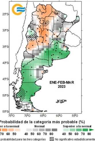
Pronóstico de Precipitación (Modelo 1)
