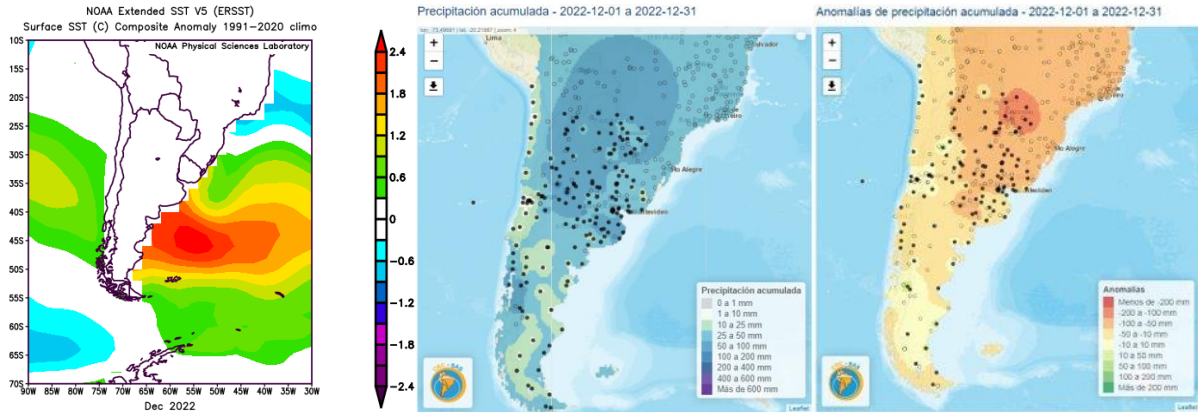
FIG. 8 –Anomalías de la temperatura superficial del diciembre de 2022. Período de referencia 1991-2020. Fuente: NOAA. Precipitación acumulada (centro) y anomalía (derecha) (mm) – diciembre 2022– Fuente: CRC-SAS
