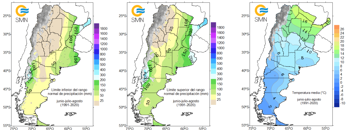
FIG. 9 – Límite inferior del rango normal (mm) (izquierda), límite superior del rango normal (mm) (centro) y temperatura media normal ( ^{\circ}\text{C} ) (derecha) para el trimestre junio-julio-agosto. Período de referencia 1991-2020.
