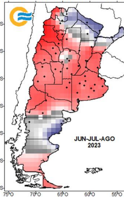
Probabilidad de la categoría más probable (%)
