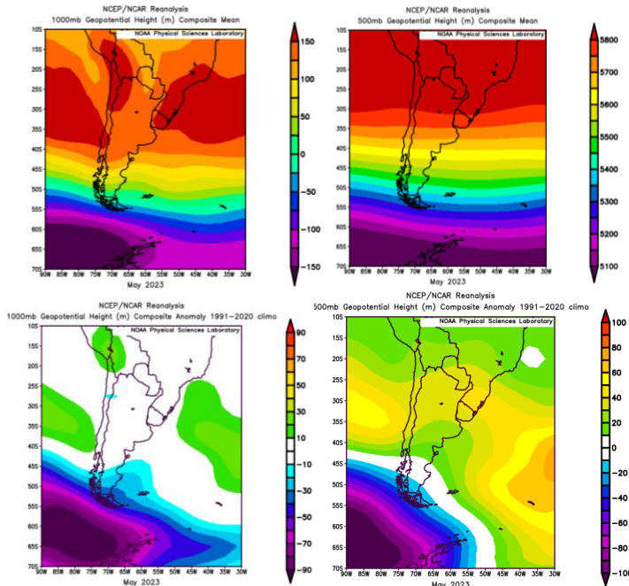
FIG.7– Campo medio de altura geopotencial de la superficie isobárica de 1000 y 500 hPa (arriba) (m) y anomalía (abajo) mayo de 2023
