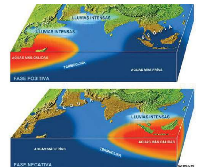
Esquema de las fases positiva y negativa del Dipolo del Océano Índico. Fuente: WHOI (Institución Oceanográfica de Woods Hole) - MetEd-COMET Program (Programa Cooperativo para Meteorología Operativa, Educación y Entrenamiento)
