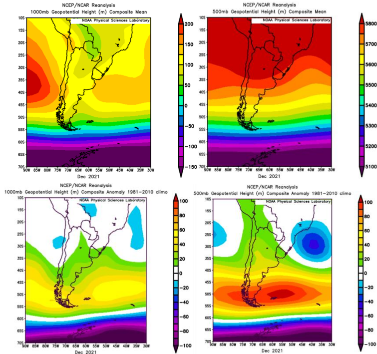
FIG.7– Campo medio de altura geopotencial de la superficie isobárica de 1000 y 500 hPa (arriba) (mgp) y anomalía (abajo) diciembre 2021
