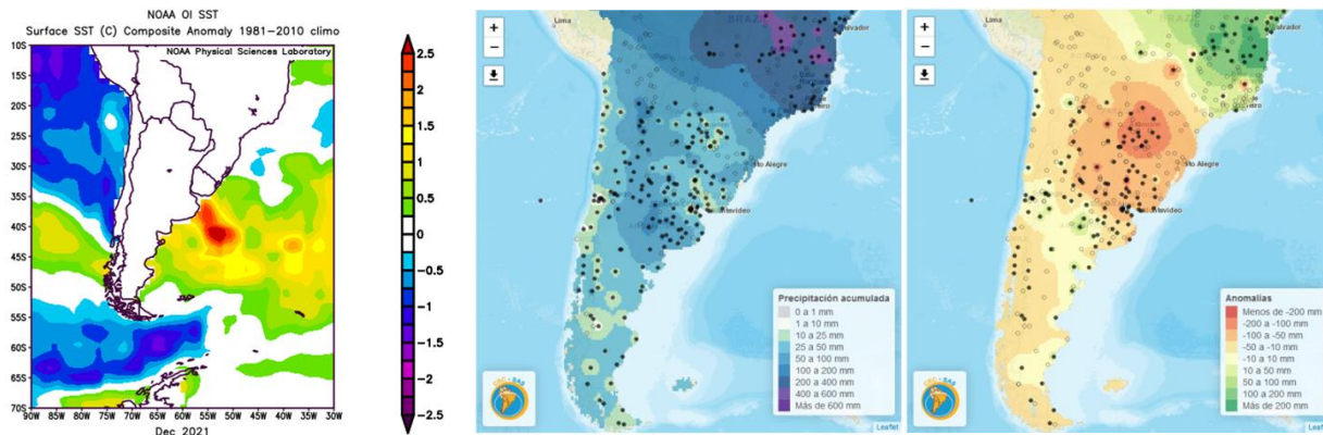
FIG. 8 –Anomalías de la temperatura superficial del mar diciembre 2021. Período de referencia 1981-2010. Fuente: NOAA. Precipitación acumulada (centro) y anomalía (derecha) (mm) – diciembre 2021– Fuente: CRC-SAS
