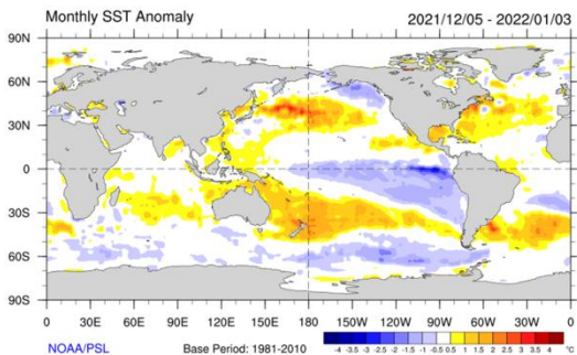
Figura 1 - Anomalías de la temperatura superficial del mar de diciembre de 2021. Período de referencia 1981-2010. Fuente: NOAA-CIRES/CDC
